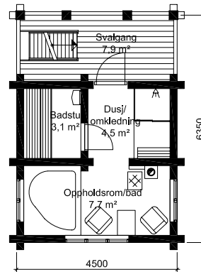
Plan 2.etg.
